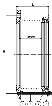
Тип 1 Type 1
