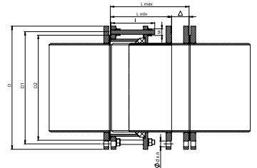
Тип 2 / Type 2
