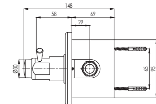
Armatura samozapiralna Slavina samozatvarjuća Self closing mixer
