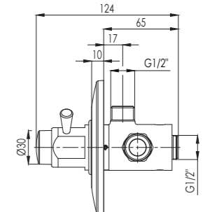
Armatura samozapiralna Slavina samozatvarjuća Self closing mixer
