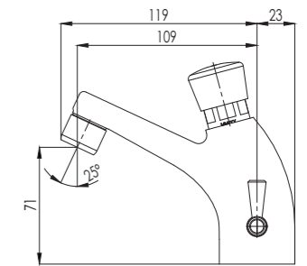
Armatura samozapiralna Slavina samozatvarjuća Self closing mixer
